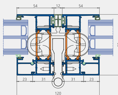
Horizontale doorsnede
