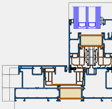
Verticale doorsnede (duorail)
