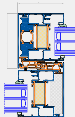
Horizontale doorsnede
